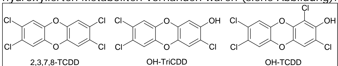
Abbildung: TCDD und die beiden erstmals beim Menschen nachgewiesenen Metaboliten 2,3,7-Trichloro-8-hydroxydibenzo-p-dioxin (OH-TriCDD) und 1,3,7,8-Tetra-chloro-2-hydroxydibenzo-p-dioxin (OH-TCDD)
